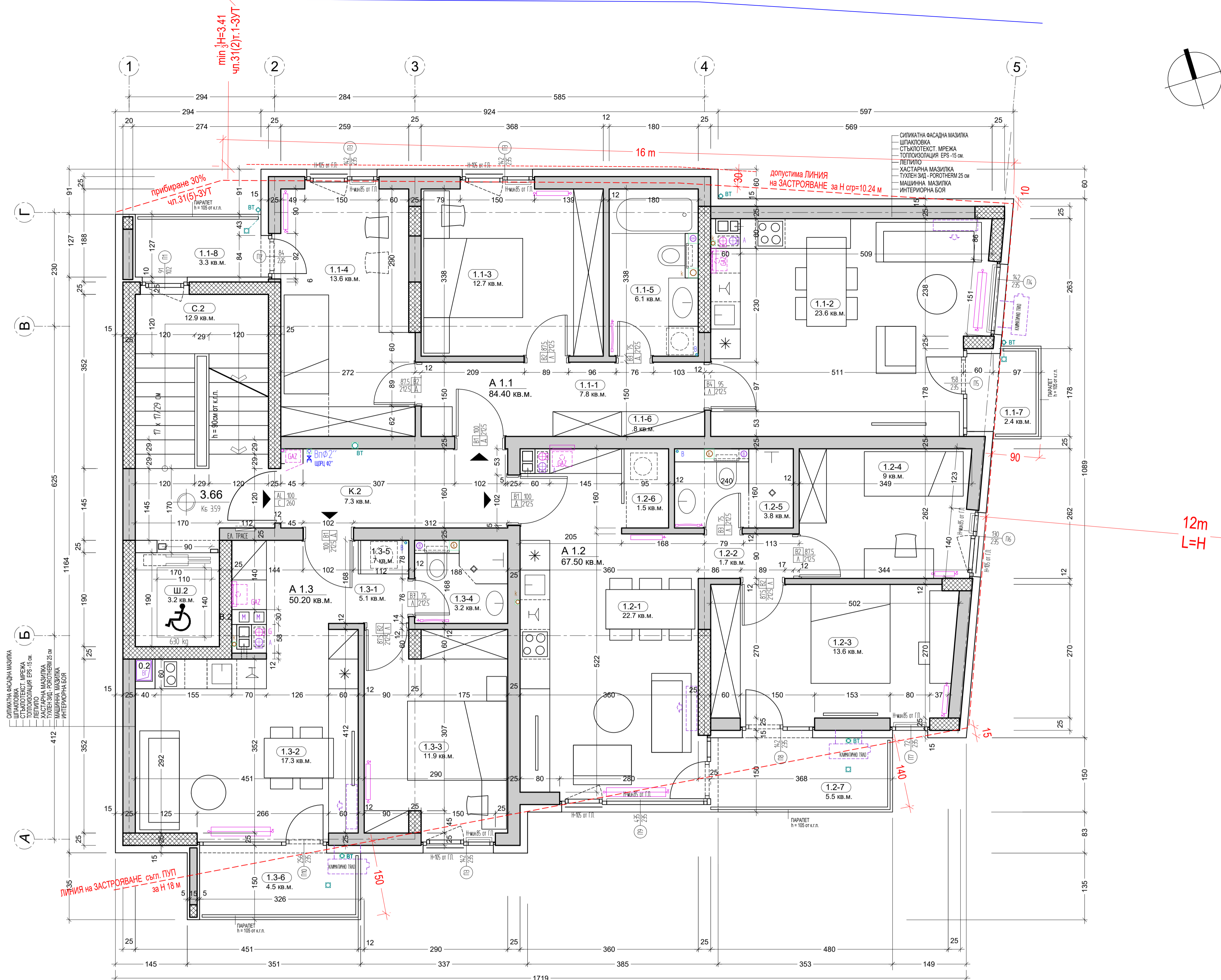
ЕТАЖ ВТОРИ - ЖИЛИЩЕН ЕТАЖ 1 ЗАСТР. ПЛОЩ НА ЕТАЖА [кв.м] 233.80
